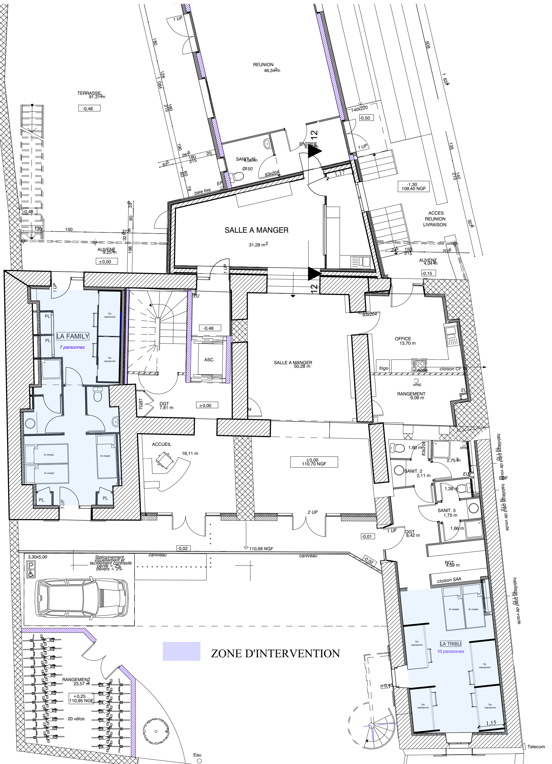
VUE EN PLAN RDC - GENERALE
